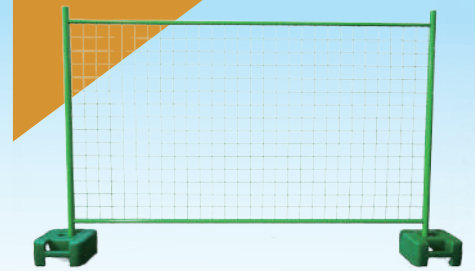
品名：全網/丙種圍籬/方形 規格：1.2x1.8m/點焊 料號：CX0118
